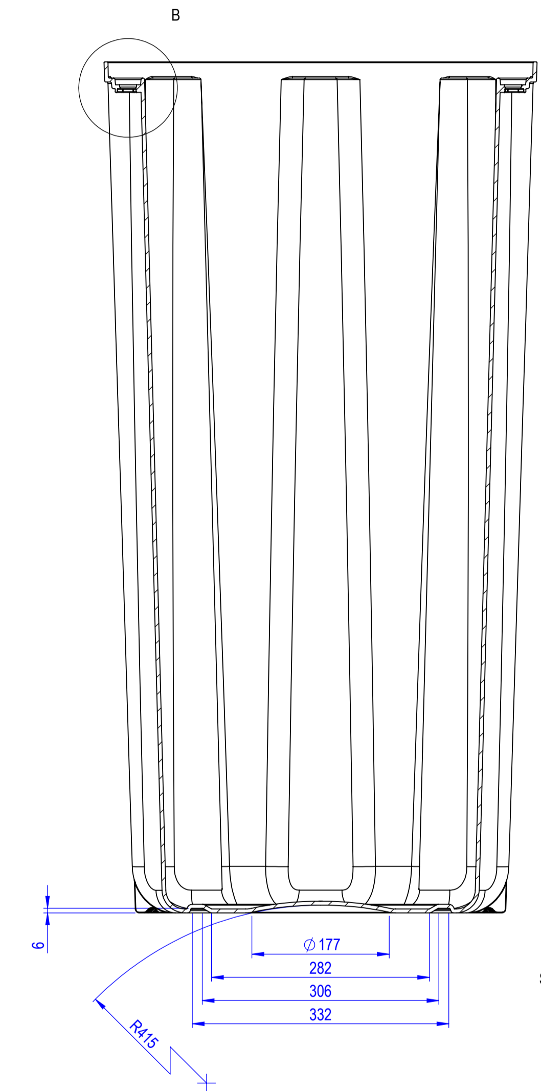
SECTION A-A
